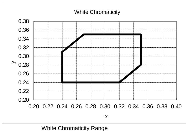
【White Chromaticity Range】
