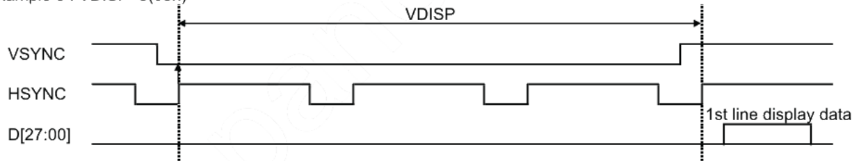
Example 3 : VDISP=3(03h)
