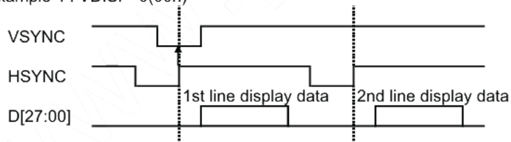
Example 4 : VDISP=0(00h)
