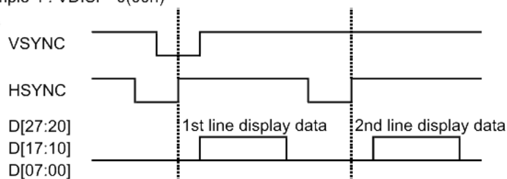
Example 4 : VDISP=0(00h)
