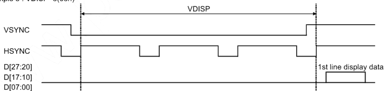
Example 3 : VDISP=3(03h)
