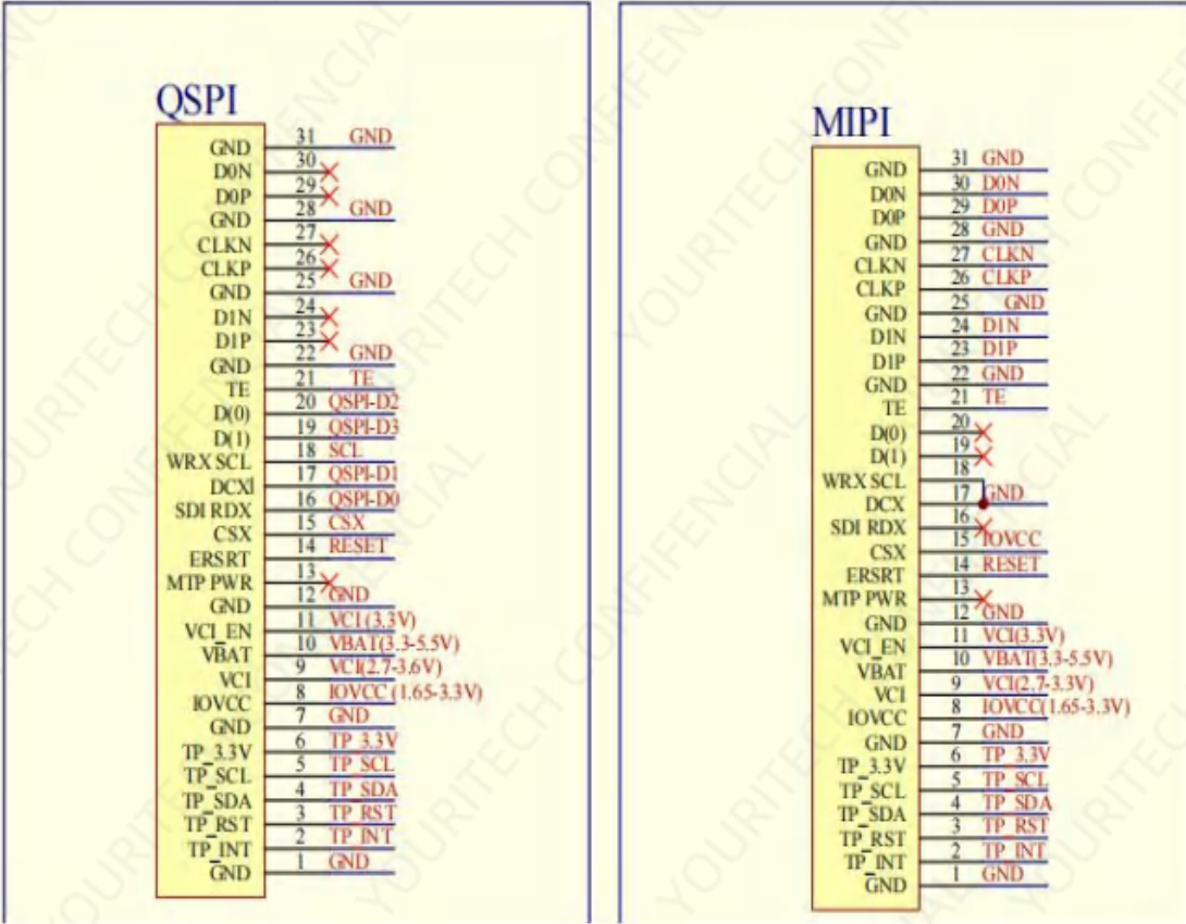
QSPI接口参考接线图
