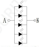
5 灯并联 2.9~3.2V 100mA
