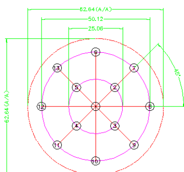
13 点均一性管控测试点
