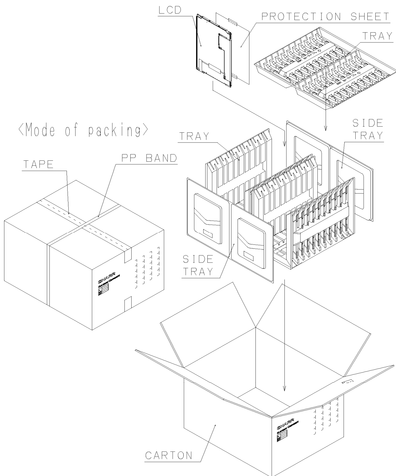
图3. 包装形态图
