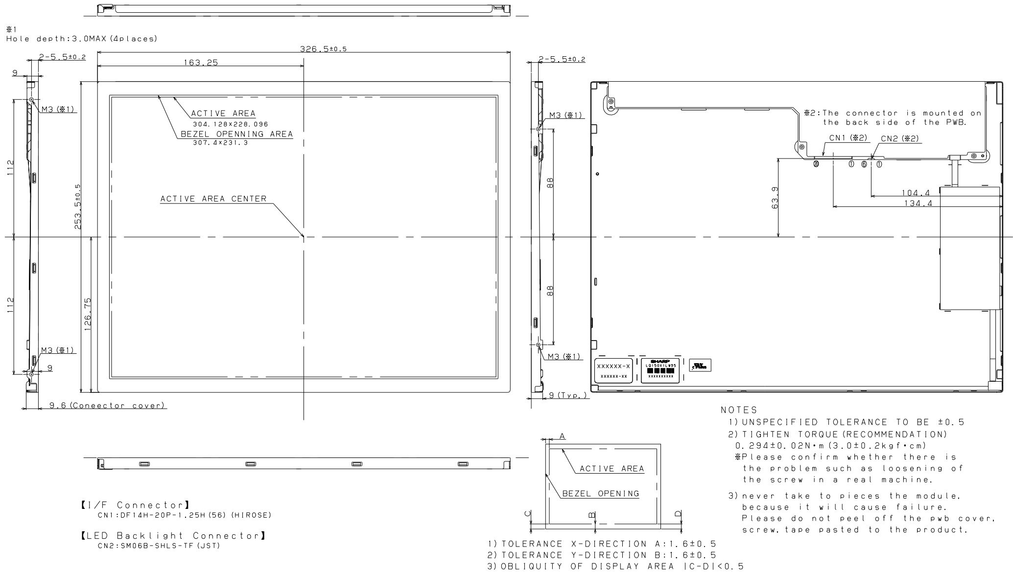
图1. LQ150X1LW95外形尺寸图 Fig.1. Outline Dimensions
