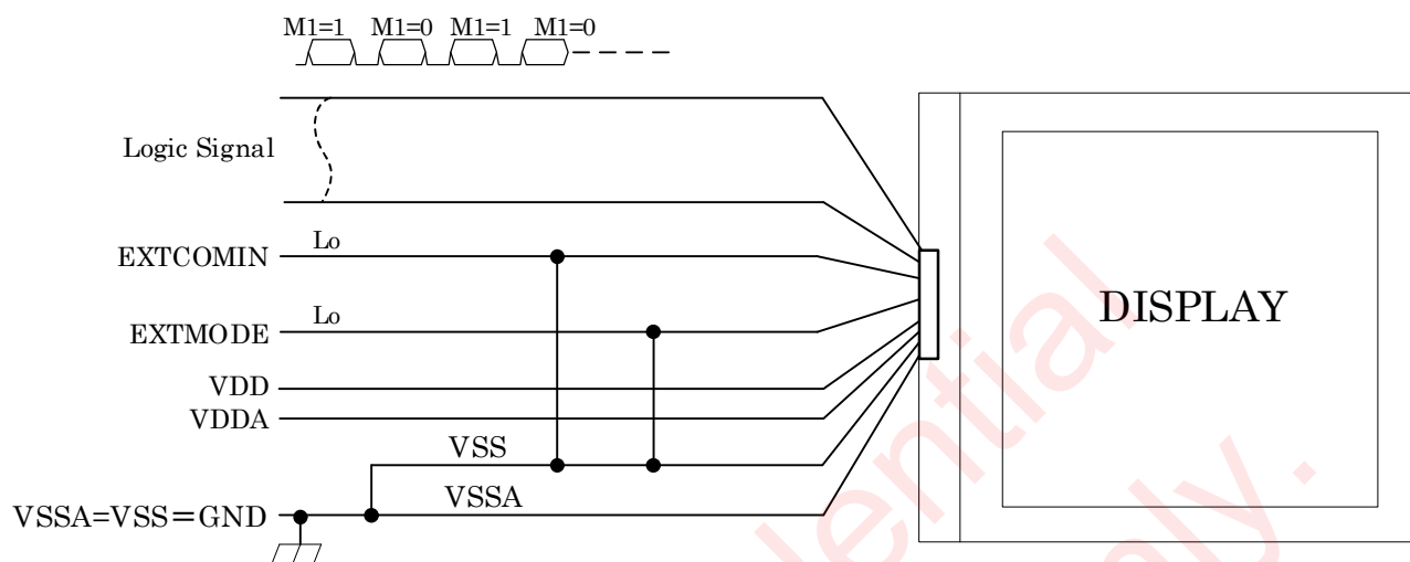
&lt; EXTMODE="Lo"&gt; COM Signal Serial Flag Input
